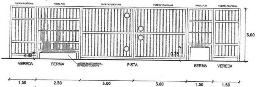
ELEVACION OPC.3
