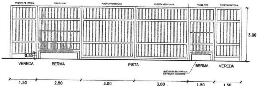
ELEVACION OPC.1
