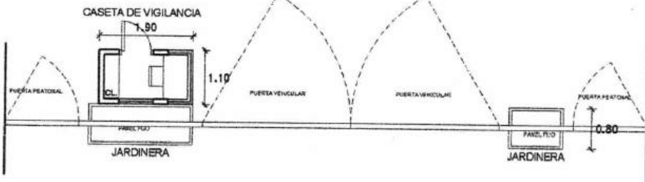
PLANTA
