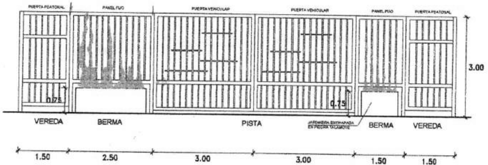
ELEVACION OPC.2
